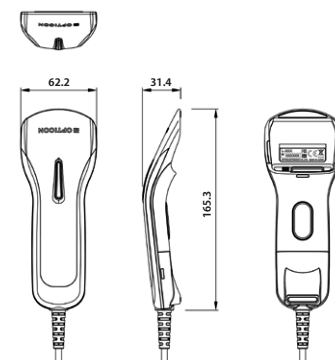
■ 外形寸法図
